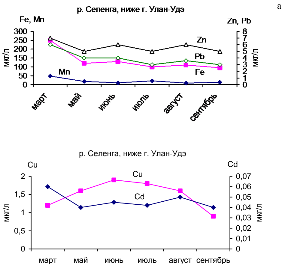
Рис. 6. Сезонное изменение растворенных форм металлов Fe, Mn, Zn, Pb (а) и Cu, Cd (б) в реке Селенга ниже г. Улан-Удэ, 2006 г.
